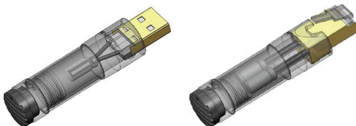
● NCF Clear Line USB/LAN的內部結構圖，由於RJ45的線路股數是USB的兩倍，因此用上了兩顆電解電容來進行雜訊消除。
